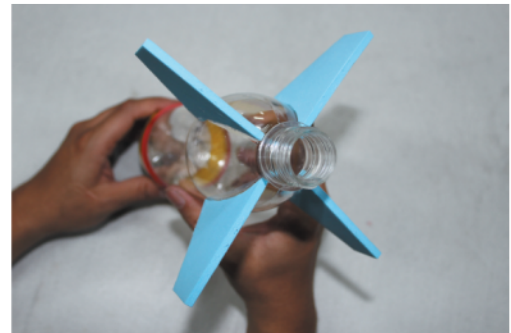
8. 將共四片EVA尾翼板平均位置黏貼處理。
